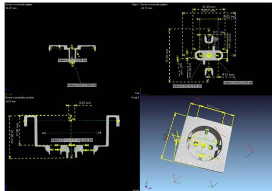
3D Vollvermessung
