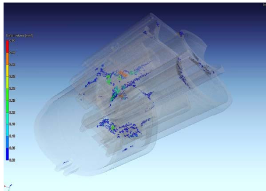
Struktur Analyse
