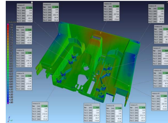
3D Soll / Ist Vergleich
